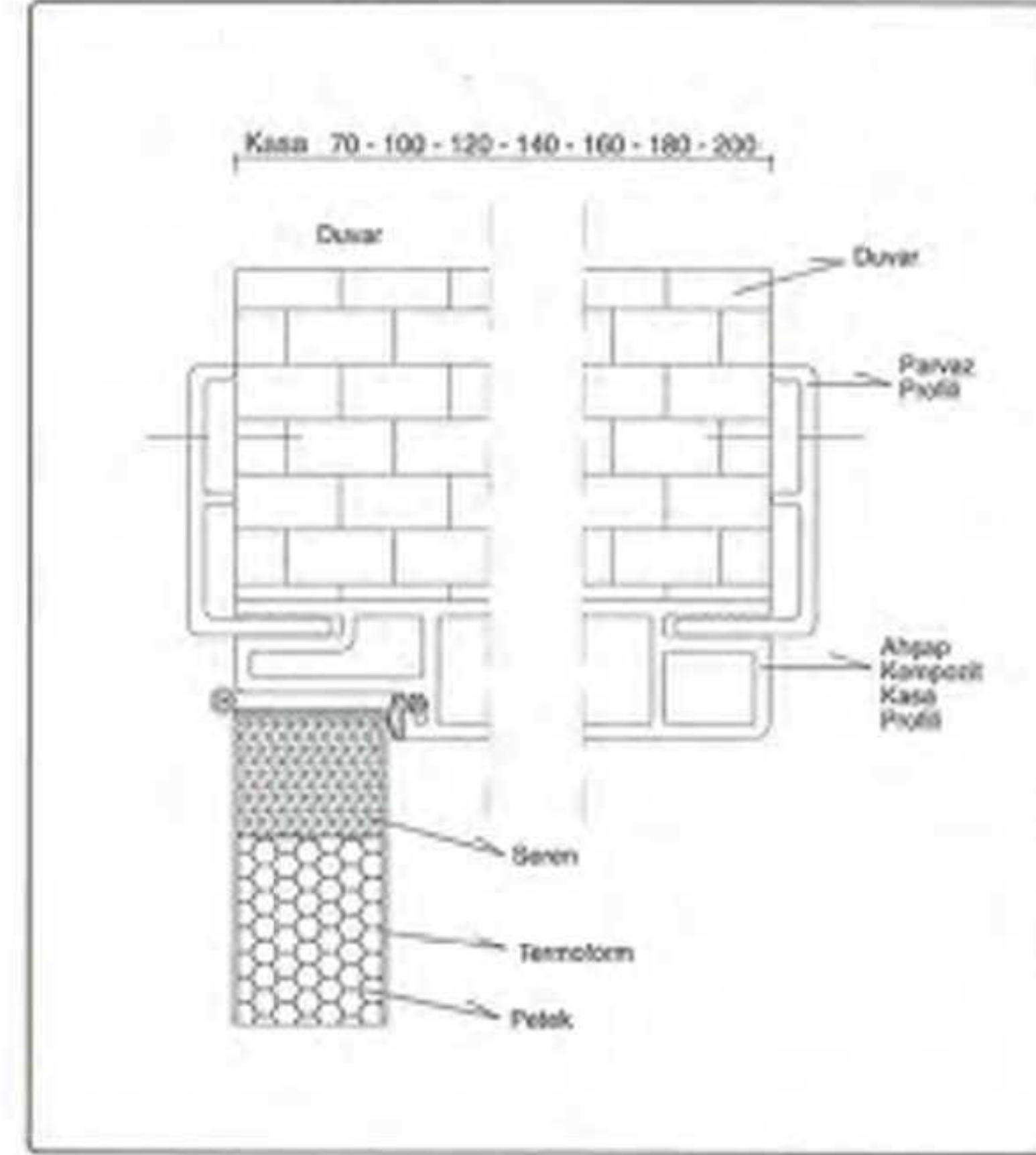
Kapı - Kasa Bağlantı Detayı Üst Ölçek 1 / 1
