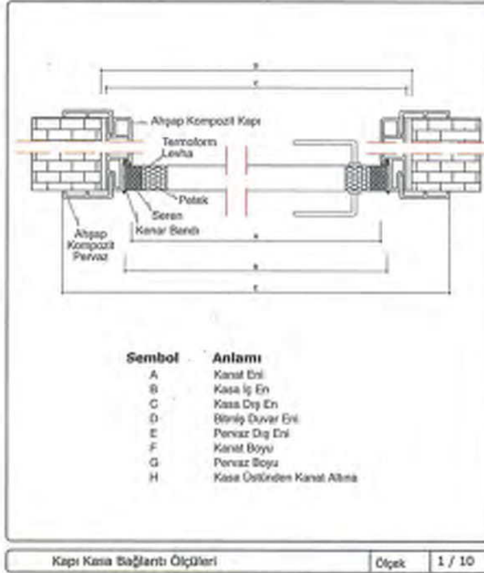
Kapı Kesit Ölçek 1 / 10
