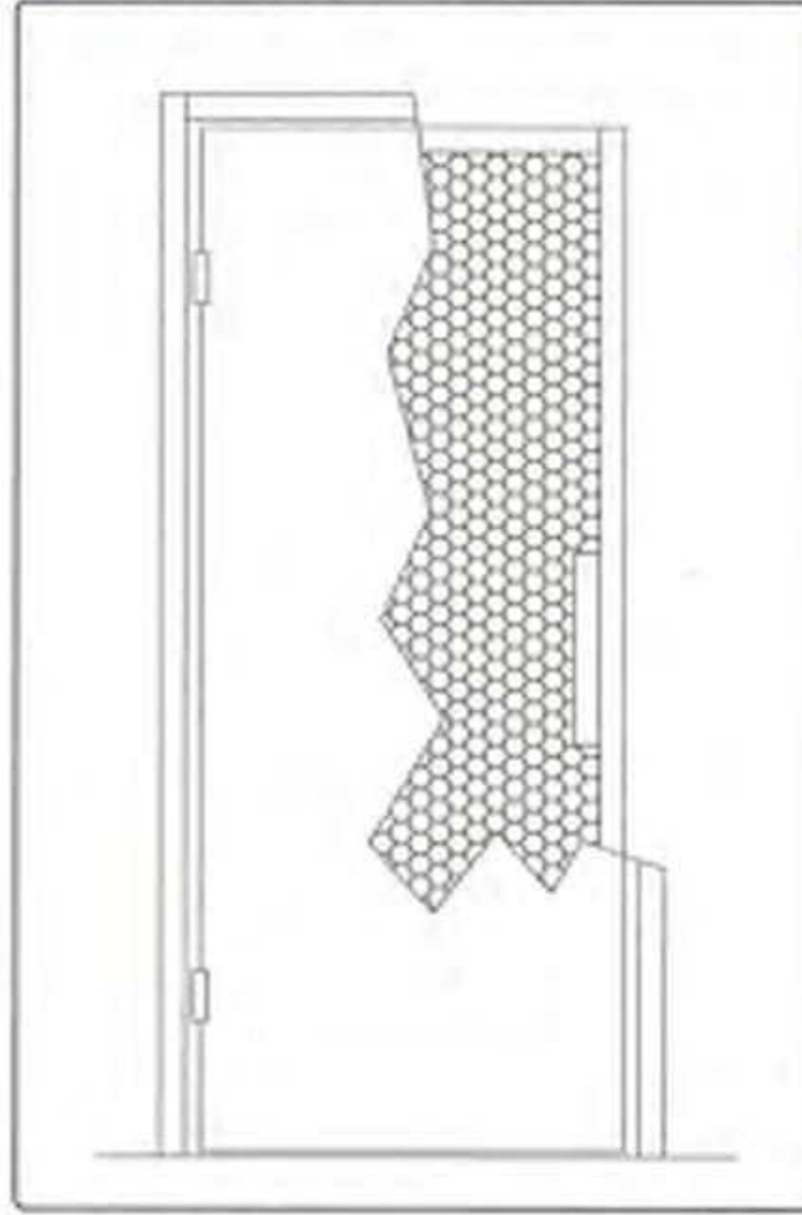
Kapı Kesit Ölçek 1 / 10
