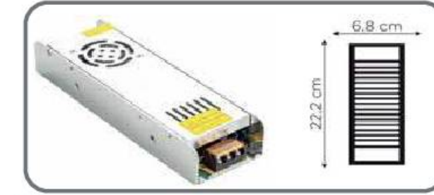
40A 500W SLIM POWER SUPPLY TRAFÖ
