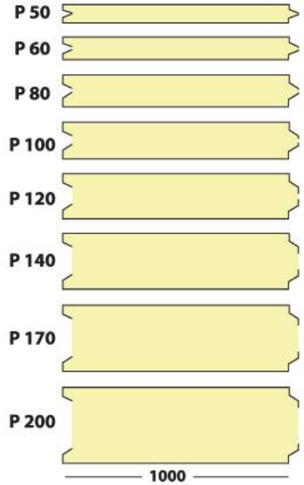
Panel Kalınlıkları Panel Thickness
