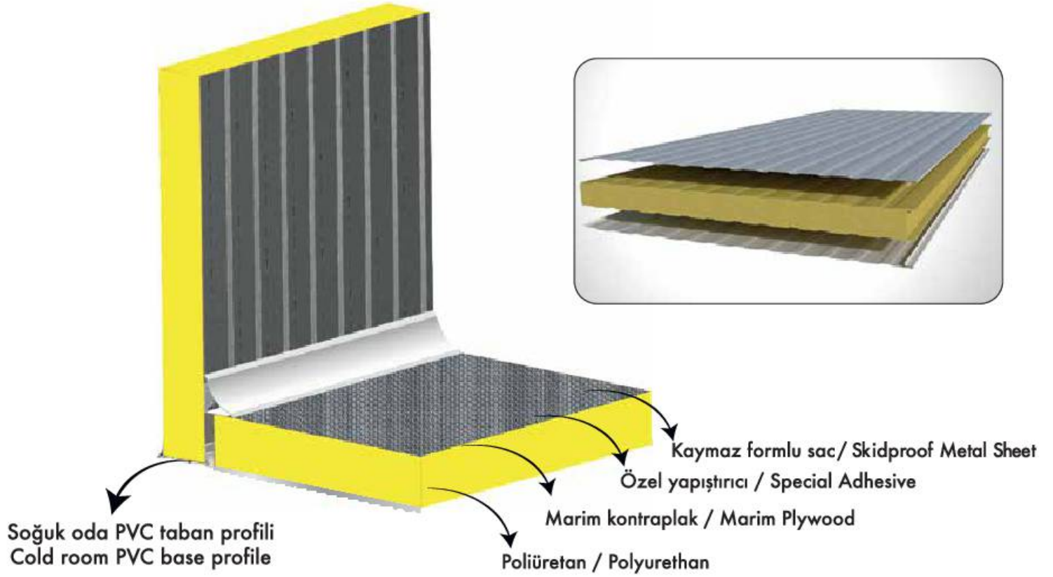
Panel Kalınlıkları Panel Thickness
