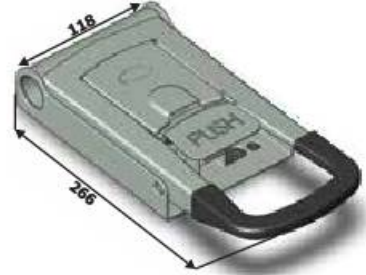
Küçük Dıştan Kilit Small External Lock
